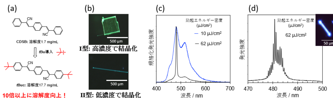
図 1 (a) 本論文での分子デザイン (b) 得られた結晶の蛍光顕微鏡像 (c) 発光スペクトルの励起エネルギー密度依存性 (d) II 型結晶から得られたレーザー発振スペクトル。挿入写真は、レーザー発振下での結晶の蛍光像。
